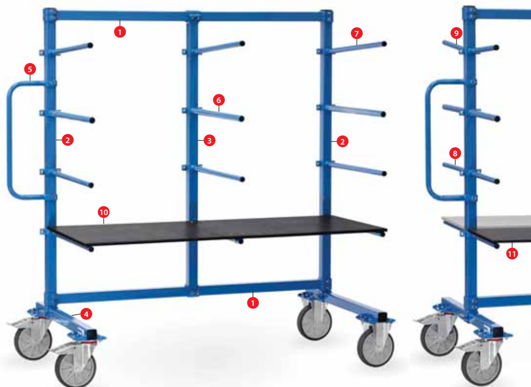
Onderdelen voor Draagarmwagen
